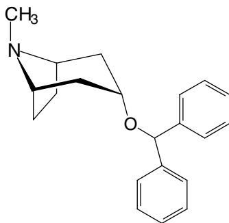
(19) Benztropine
