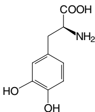
(3) LDOPA
