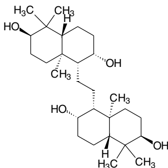
(67) Lyclavatul
