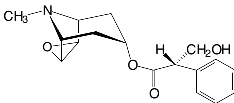
(18) Hyoscine
