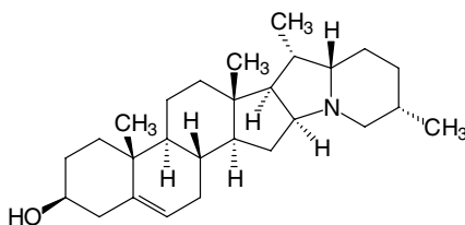
(50) Solanidine
