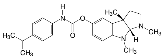
(37) Cymserine
