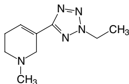
(31) LU 25-109
