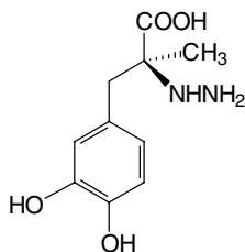
(4) Carbidopa
