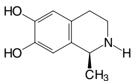
(17) Salsolinol
